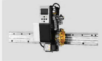
自动换底线装置
